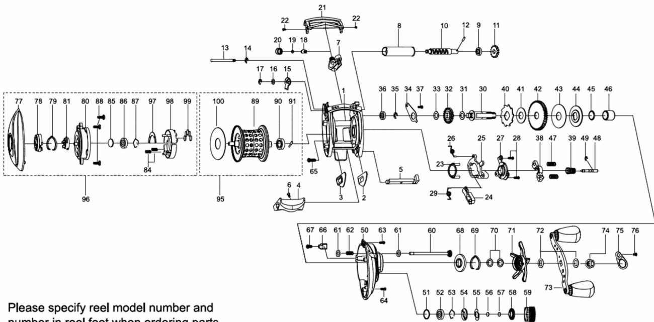
Ambassadeur REVO LTX 2100
